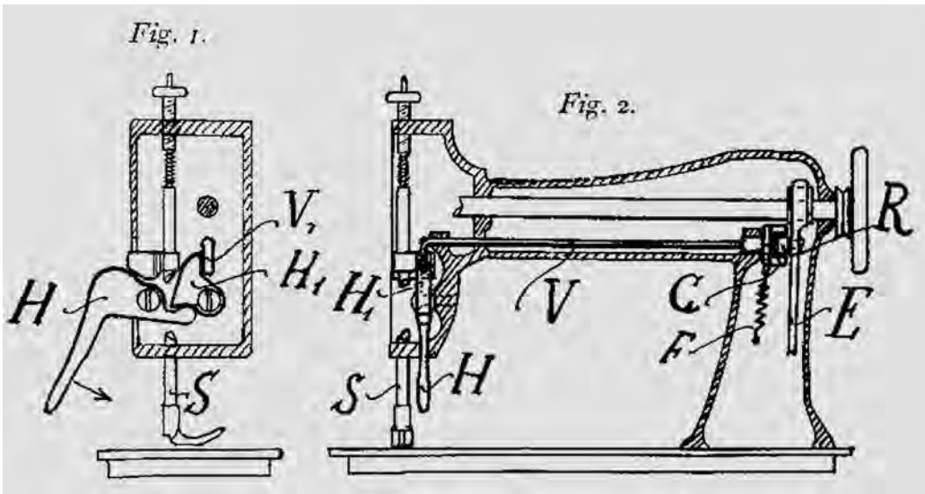
Drittes Reichspatent von Christian Hahn.
