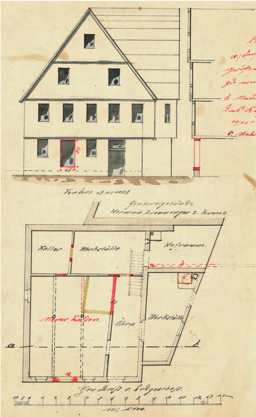
Baugesuch von Christian Hahn von 1887.
