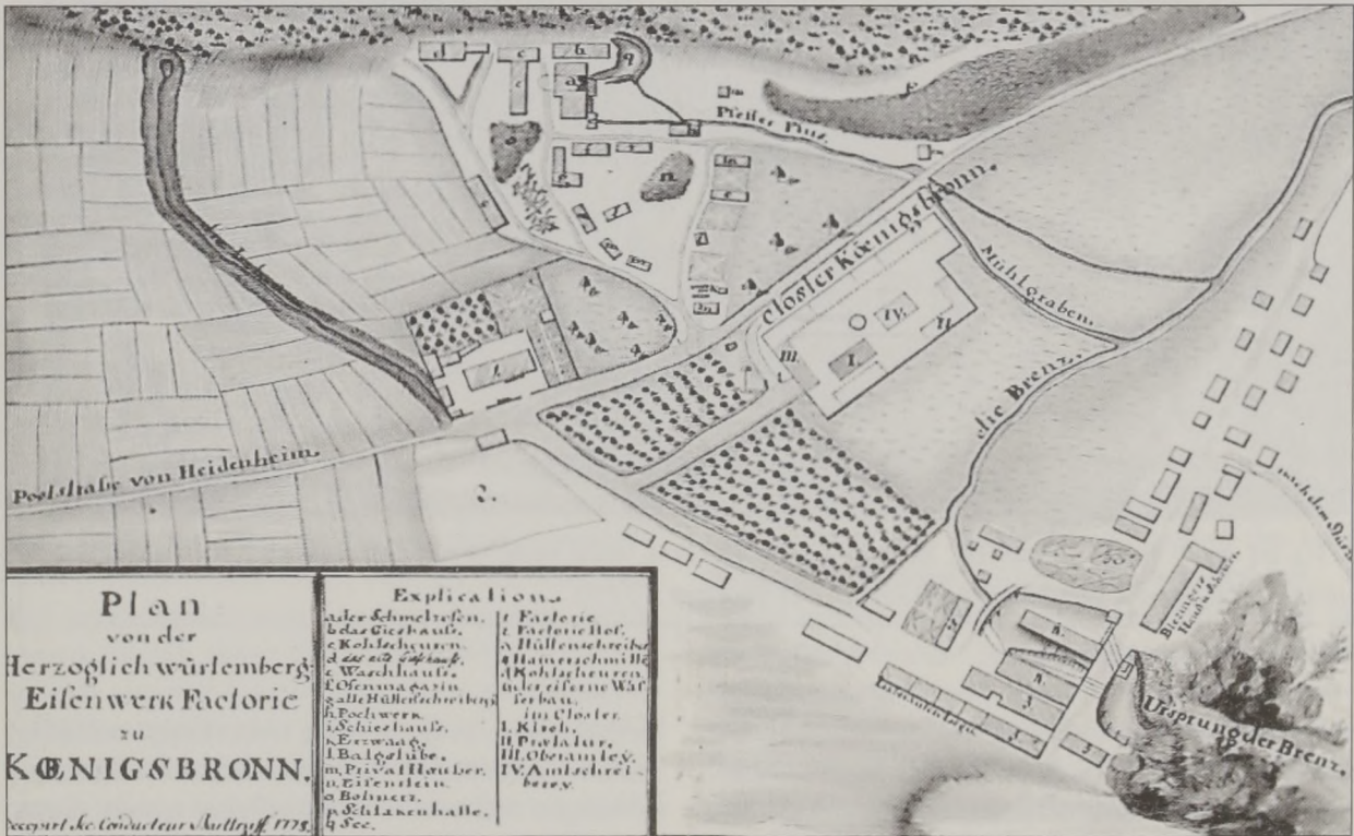
Lageplan der „Herzoglich württembergischen Eisenwerk Factorie zu Königsbronn“ aus dem Jahr 1778.
