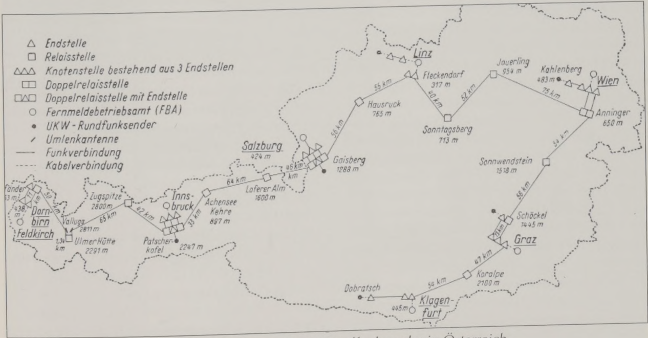
Richtfunknetz zur Programmversorgung der UKW-Rundfunksender in Österreich.
