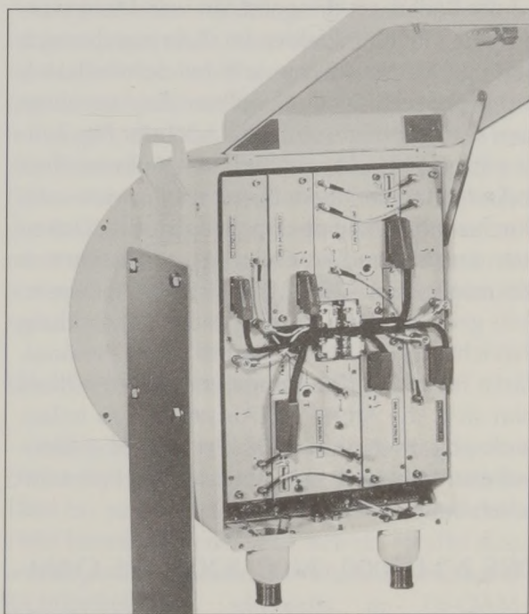
Blick in ein geöffnetes Wetterschutzgehäuse des DRS 2-140/18700.
