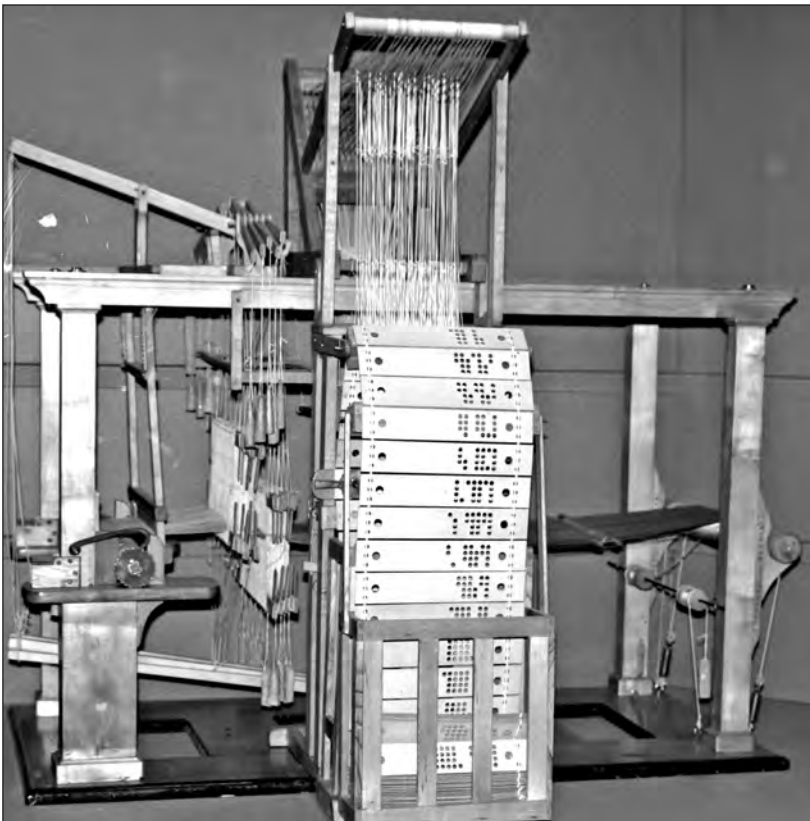
Modell eines mit Lochkarten gesteuerten Jacquardwebstuhls.
