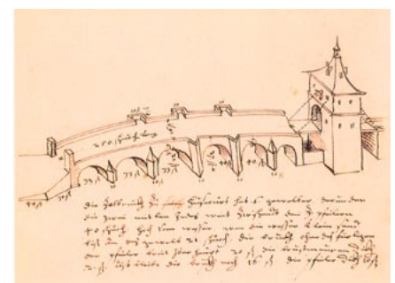
Die Zollbrücke von Voujeaucourt. Federzeichnung von Heinrich Schickhardt
