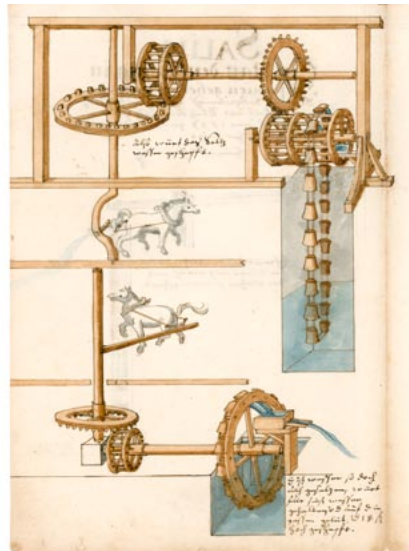
Salzwerk Salins in Burgund. Kolorierte Zeichnung des Paternosterwerks von Heinrich Schickhardt, 1593
