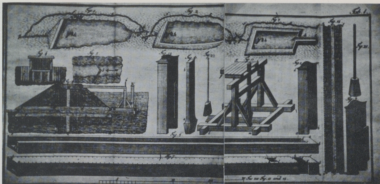
Abb. 12 Zeitgenössische Darstellung eines Schlegels (Striegels) d. i. die Absenkvorrichtung an Teichen aus CANCRIN: Bauschriften, Marburg 1799.
