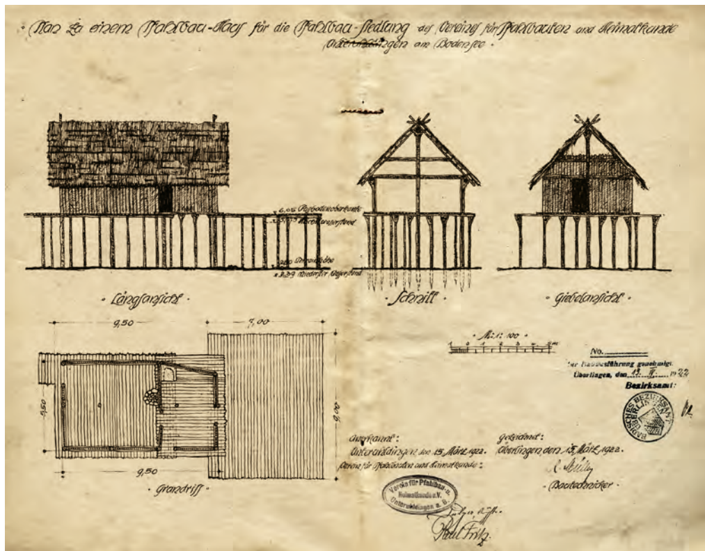
Bauplan des Architekten Paul Fritz für die ersten beiden Pfahlbauhäuser in Unteruhldingen
