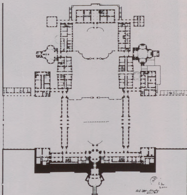
R. F. H. Fischer: Schloss Ludwigsburg. Grundriss des Erdgeschosses, Zeichnung um 1794. Der Pfeil am Rand deutet auf die Schlosskapelle.
