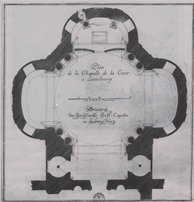
D.G. Frisoni: Schlosskapelle Ludwigsburg, Grundriss.
