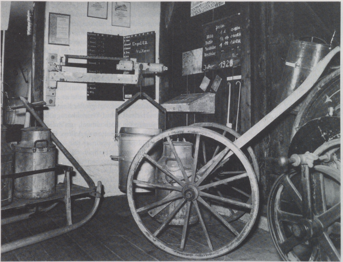
Milchannahme: Waage, Schreibpult und Anschreibtafel sowie Fahrzeuge zur Milchlieferung.
