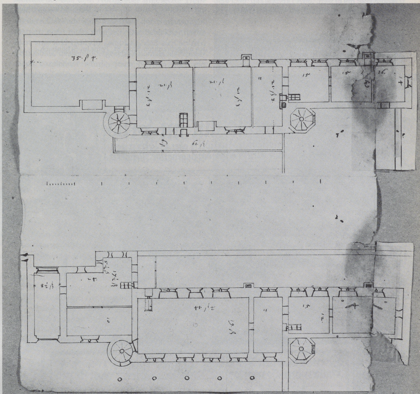
Abb. 3 Pläne des Schloßchens von Heinrich Schickhardt, 1619. Unten: Erdgeschoß, oben: Obergeschoß. (Foto: Hauptstaatsarchiv Stuttgart)
