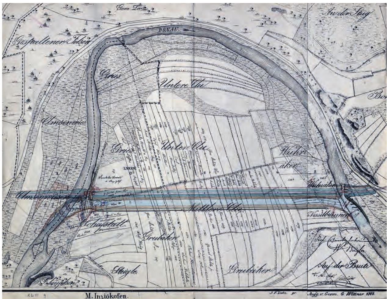
Beim Bau der Donautalbahn wurde im Bereich Untere Au bei Laiz die Donau auf einer Länge von 700 Metern verlegt. Im Plan ist die Zerschneidung der Grundstücke, die aufgrund eines preußischen Gesetzes für den Bahnbau enteignet wurden, deutlich zu erkennen.
