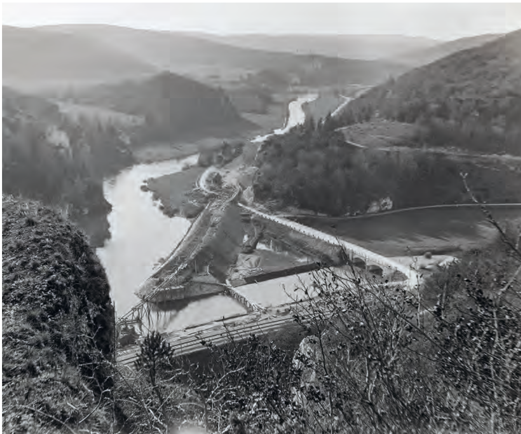
Der Bau der Brücke an der Schmeiemündung war risikoreich, musste mit einfachen Holzgestellen begonnen werden, und ein hoher Bahndamm war nötig. Im Vordergrund die Bahnlinie Tübingen, die bereits seit 1878 bestand; in der Bildmitte die neue Straßenführung mit dem Durchbruch des Bahndamms.
