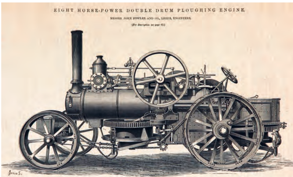
Dampfflug aus einem Prospekt von John Fowler in Leeds (1896). Da die Dampfmaschinen viel zu schwer für einen feuchten Acker waren, wurde der eigentliche Pflug zwischen zwei Maschinen an einem Drahtseil über den Acker gezogen.
