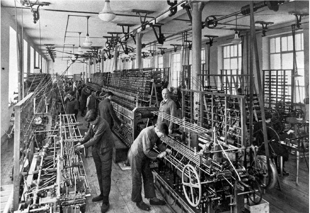
Abb. 3 - Seideplattier- und Häkelgalonmaschinen, Posamentenfabrik Gustav Gerster, Biberach, 1928.
