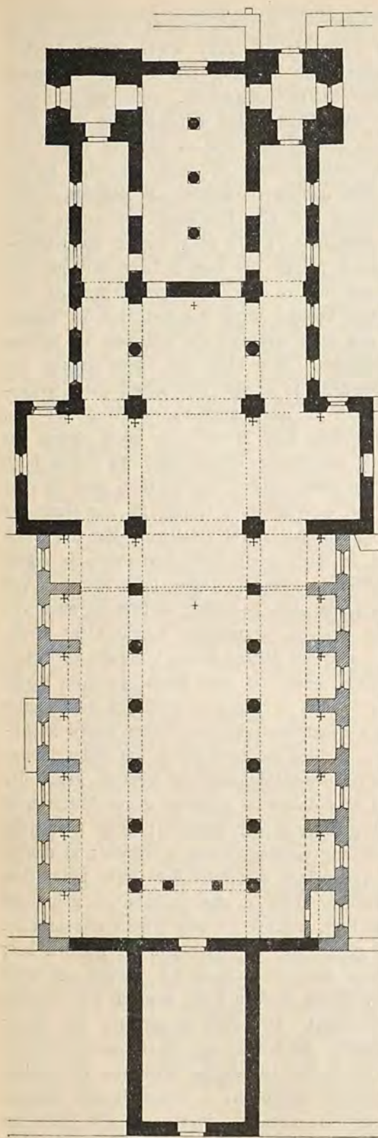
Grundriß des alten Münsters.
