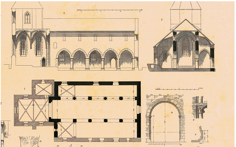
Querschnitt und Grundriss der Johanniskirche in Brackenheim. Detailreiche Zeichnung aus dem von Eduard Paulus (dem Jüngeren) seit 1889 in mehreren Bänden und Auflagen herausgegebenen Werk Die Kunst- und Altertums-Denkmale im Königreich Württemberg. (Vorlage: Zabergäuverein)
