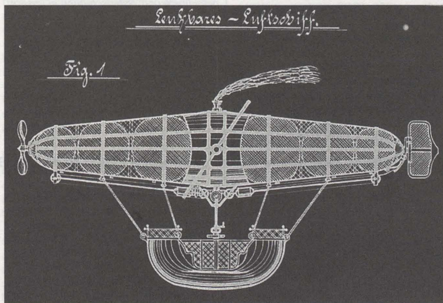
Lichtpause eines Luftschiffentwurfs des Heilbronner Mechanikers Karl Fritz, 1905. Aufnahme: Hauptstaatsarchiv Stuttgart
