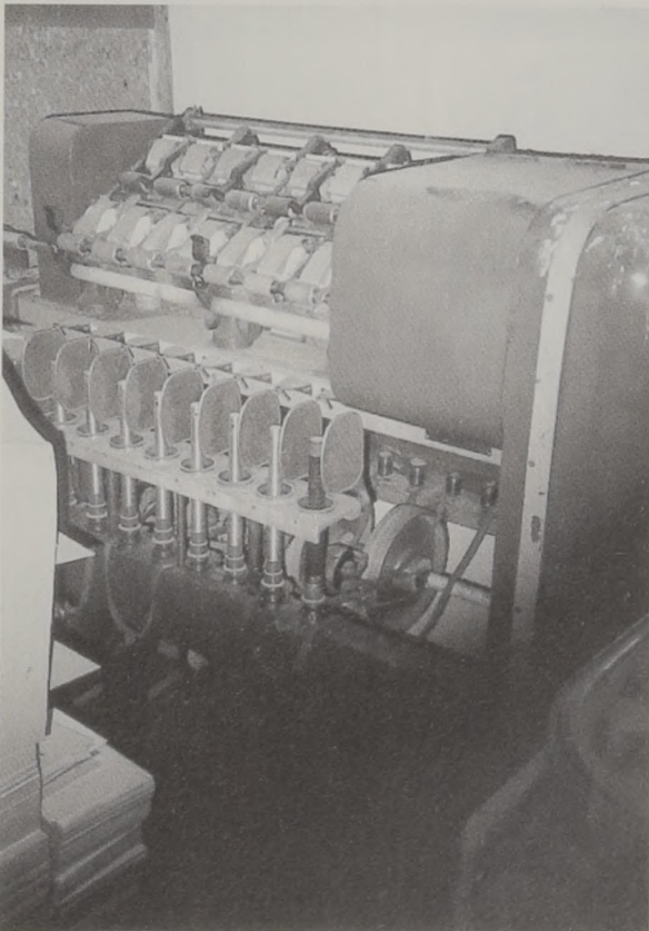
Versuchsringspinnmaschine für Baumwollgarn.
