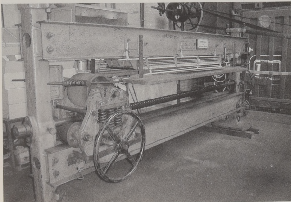
Bügel- und Narbenpressmaschine aus dem Jahr 1938.
