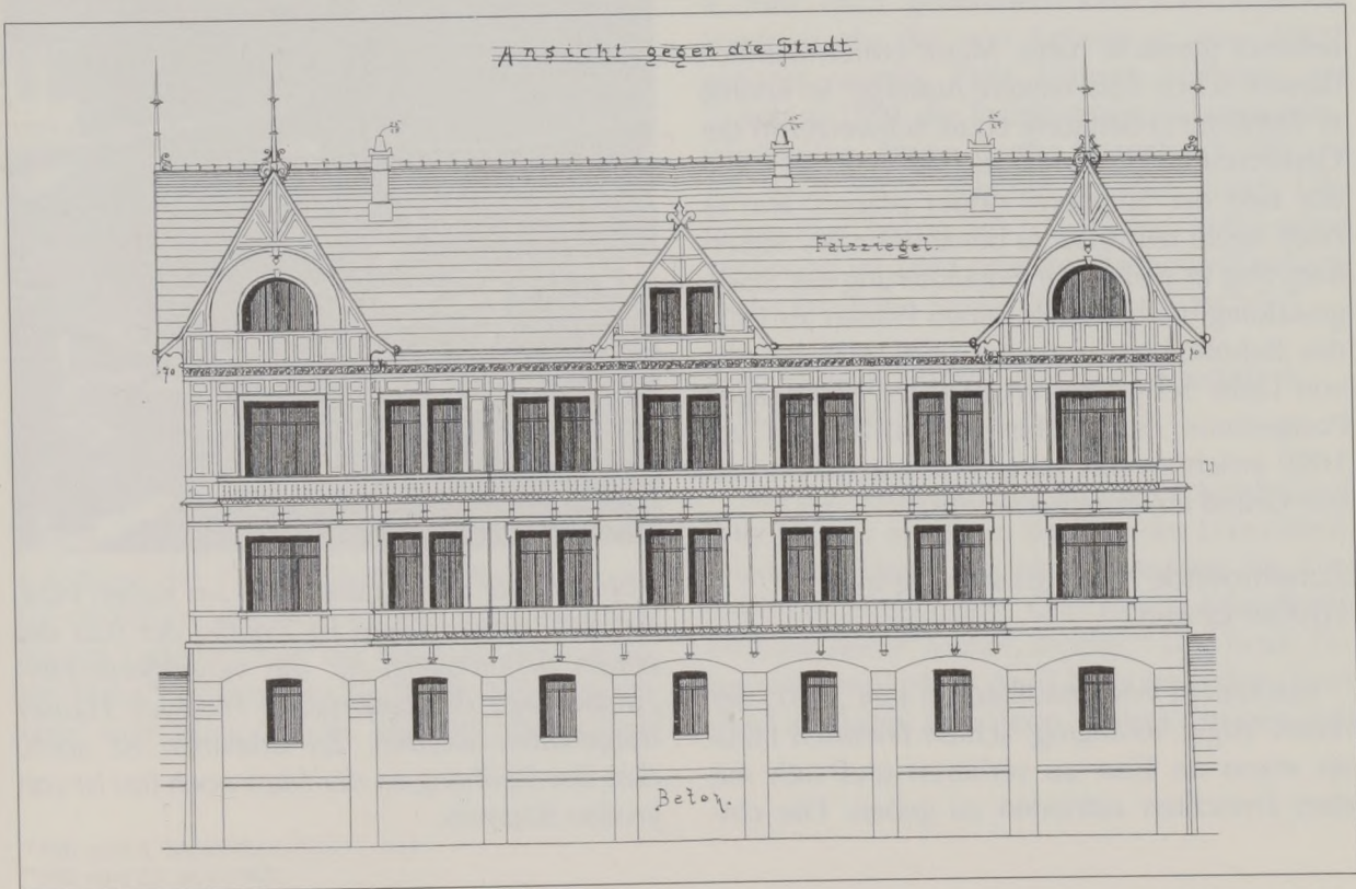
Abb. 25: Diese Bauzeichnung zeigt die von Architekt P. J. Manz vorgesehene Gliederung der Hangseite.
