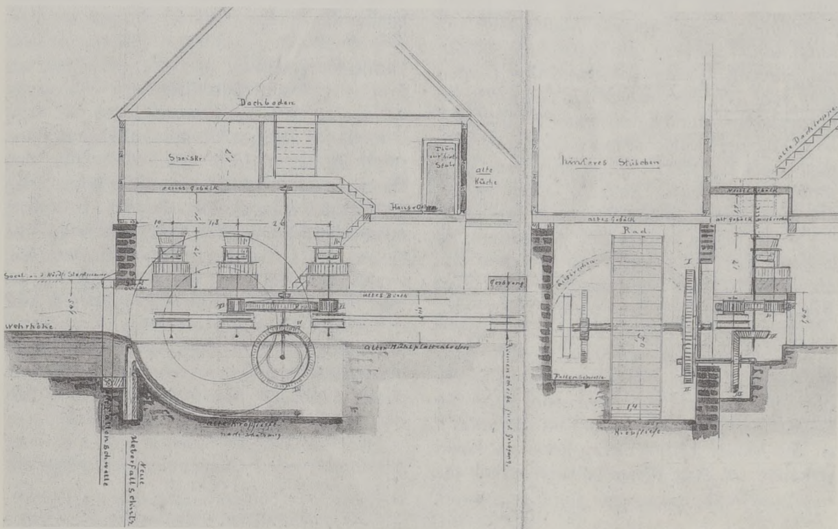
Abb. 2: Querschnitt durch die Rüflensmühle im Jahr 1878.
