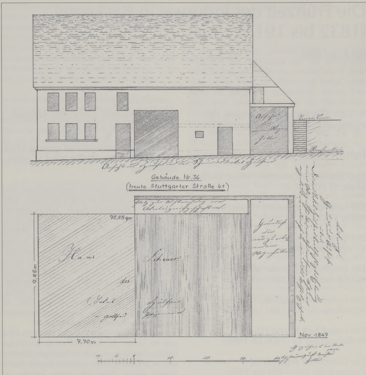
Abb. 1: Grundriss und Ansicht des dem Bauern und Fuhrmann Jakob Häuser zur Hälfte gehörenden Anwesens Nr. 36 (Stuttgarter Straße 41). Abgebildet auf einem Baugesuch für die Erweiterung der Scheuer, vom November 1847.
